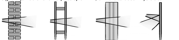
betón, tehla straty: 20 + 40% drevo, sádkartón straty: 5 + 20% železobetón straty: 40 + 90% oceľová stena straty: 90 + 100%
