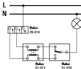
Přepínač s křížovým přepínačem
