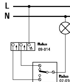
Přepínač, stmívač na straně sítě
