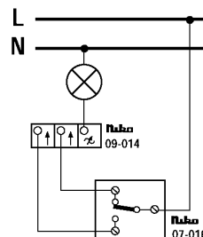
Přepínač, stmívač na straně zátěže
